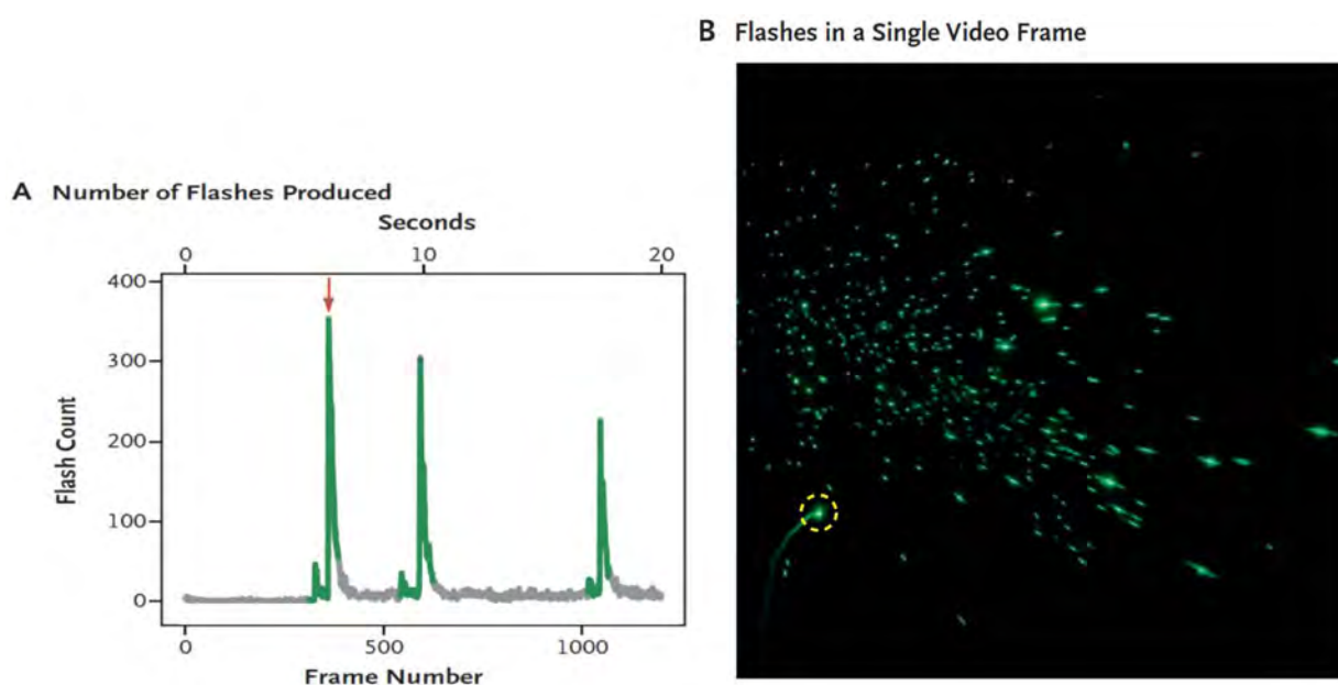
Fig. 12 Il pannello A mostra il numero dei flash registrati in un singolo fotogramma di un video con frequenza di 60 fps. Il colore verde indica l'emissione vocale. Si nota che nei periodi silenti (striscia grigia) il numero dei flash non si azzerava immediatamente, presumibilmente perché alcune goccioline permanevano nella scatola per qualche secondo. Il pannello B mostra uno dei fotogrammi corrispondente all'istante in cui l'emissione di goccioline risultava massima (freccia nel pannello A). La diversa luminosità dei flash fornisce un'indicazione della diversa dimensione della gocciolina (modificato da Anfinrud et al. , 2020).
