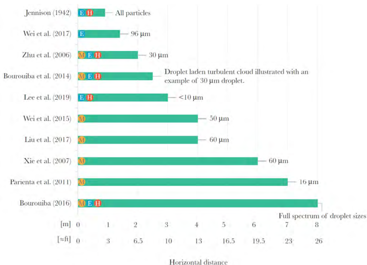
Fig. 21 Previsioni della distanza raggiunta dalle emissioni respiratorie, sulla base di modelli matematici o numerici (M), osservazioni sperimentali (E) o sperimentazione su pazienti (H): (riprodotto da Bahl et al. , 2020)
