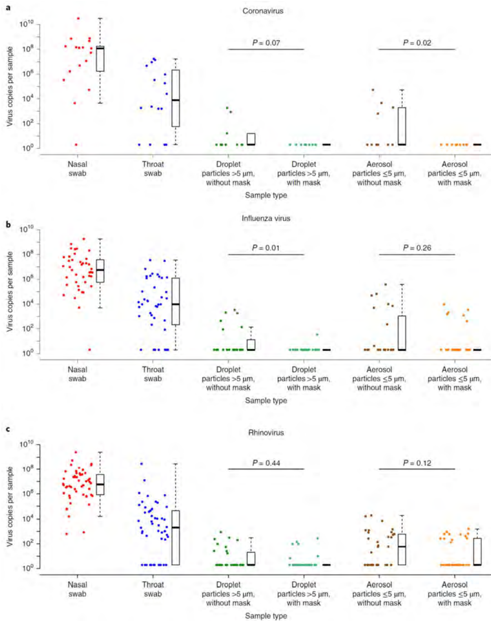
Fig. 18 Efficacia di mascherine chirurgiche nella riduzione del numero di virus respiratori emessi in gocce di taglie diverse di soggetti sintomatici affetti da coronavirus (a), influenza (b) o rinovirus (c). La Figura riporta il numero di copie per campione, raccolto attraverso tamponi nasali (rosso), tamponi faringei (blu), gocce respiratorie ( d > 5 \mu\text{m} ) raccolte per 30 min da soggetti che non indossavano (verde scuro) o indossavano (verde chiaro) una mascherina chirurgica, e particelle più piccole ( d < 5 \mu\text{m} ) raccolte per 30 min (marrone senza maschera, arancione con maschera) (riprodotto da Leung et al. , 2020).
