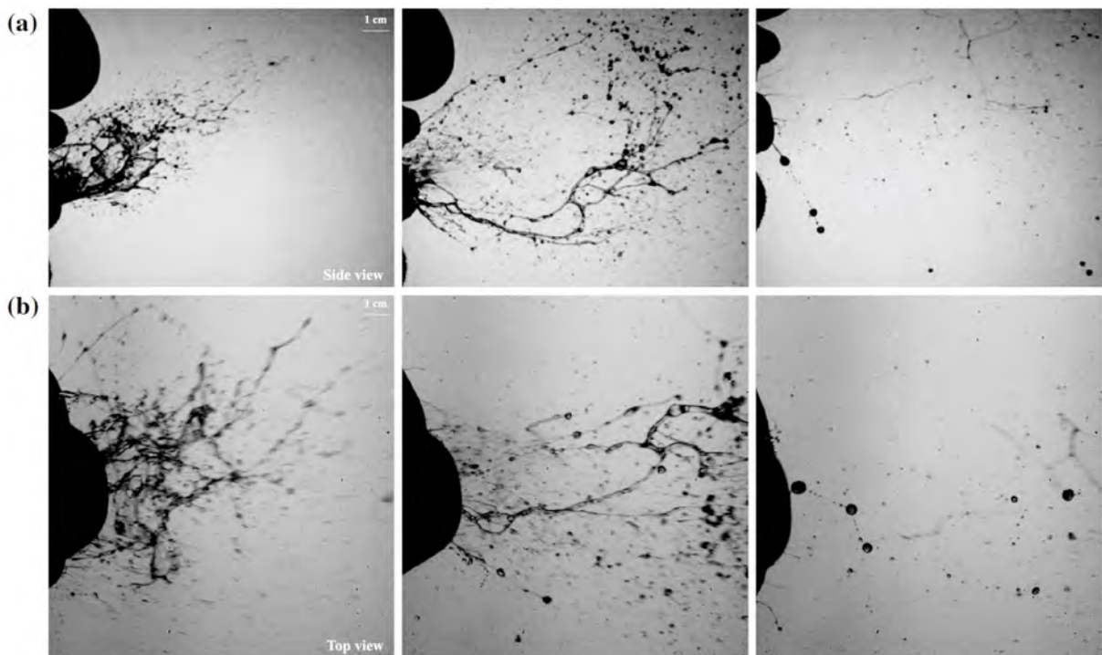
Fig. 11 La prima fase del processo di emissione associata a uno starnuto è visualizzata lateralmente (a, 8000 fps) e dall'alto (b, 2000 fps). La formazione delle gocce (colonna di destra, t=117 ms) è il risultato della frammentazione di strutture più complesse che evolvono da forme estese ( sheets and bags ) (colonna di sinistra, t=8 ms) a strutture allungate, filamenti in cui si formano i prodromi delle gocce ( pearls ) (colonna di centro, t=21 ms)
